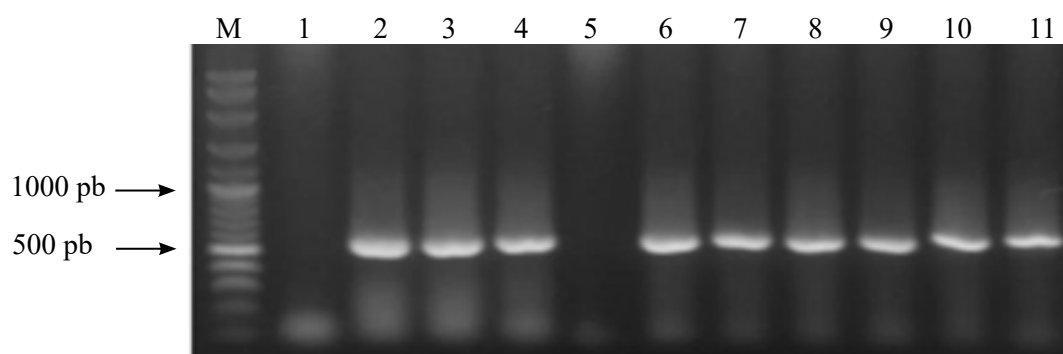
Gambar 4 Amplicon hasil PCR sampel daun kentang terinfeksi PVY. Lajur 1 = daun dari tanaman sehat; 2 = daun tanaman sakit asal Pengalengan; 3-4 = daun tanaman sakit asal Legok Bako; 5 = daun tanaman sakit asal Cipaganti; 6 = daun tanaman sakit asal Cimemyan; 7-8 = daun tanaman sakit asal Los; 9 = daun tanaman sakit asal Padaawas; 10 = daun tanaman sakit asal Kertamana; dan 11 = daun tanaman sakit asal Cimemyan.
